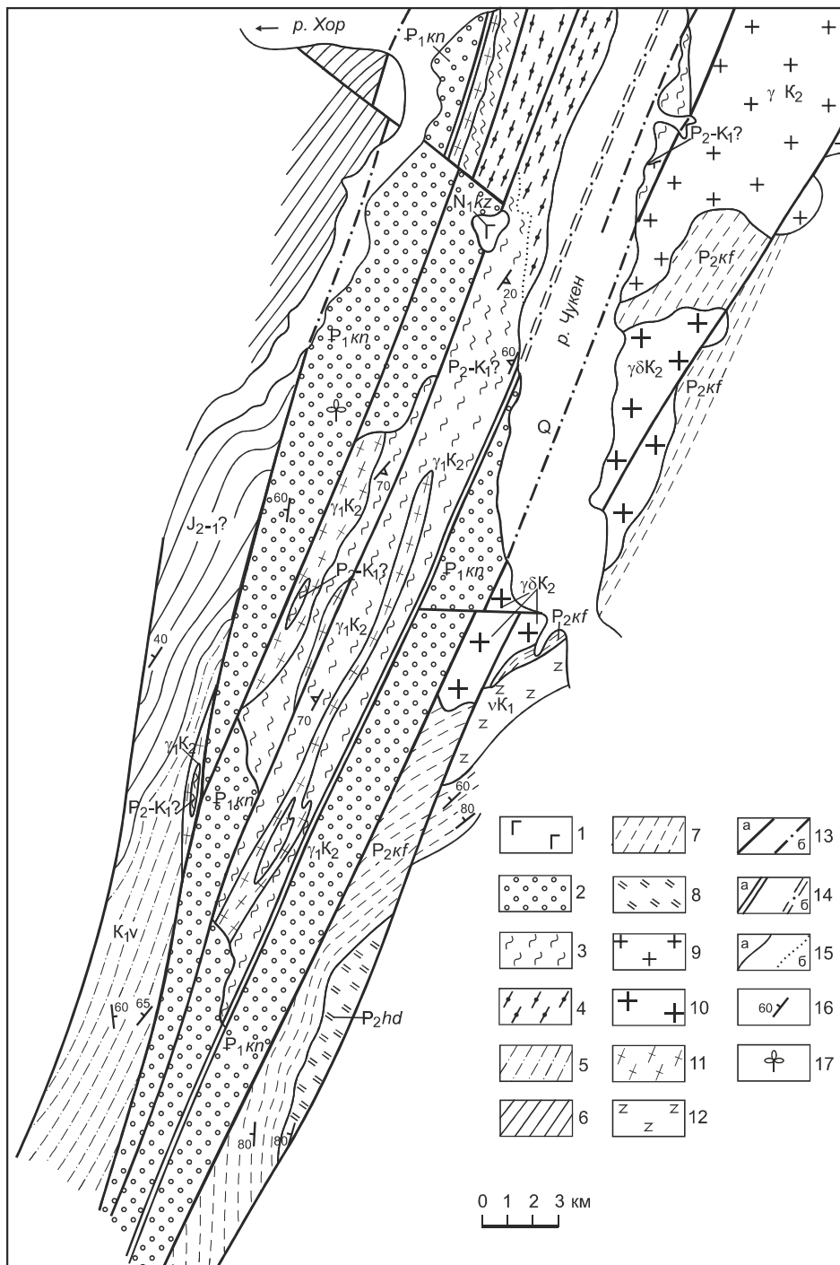
Рис. 1.8. Фрагмент геологической карты Хорского клина в зоне Центрального Сихотэ-Алинского разлома в бассейнах рр. Хор и Чуехен (В.И. Аношкин, 1978 г.)
