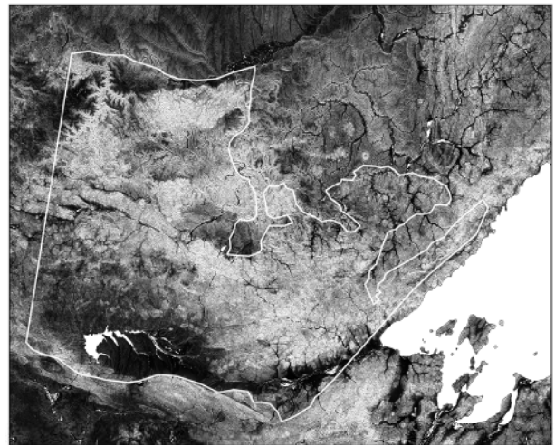
Рис. 3.1.4. ЦМР Алдано-Станового щита, обработанная оператором расчетом модуля градиента
