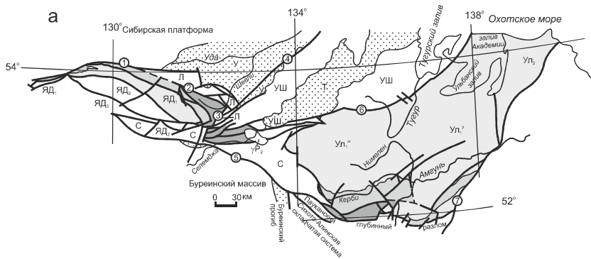
Рис. 3.4.2. Реконструкция структуры Ульбанского синклиория для конца юрского периода (б). а – современная структура района, по В.Ю. Забродину [39].
