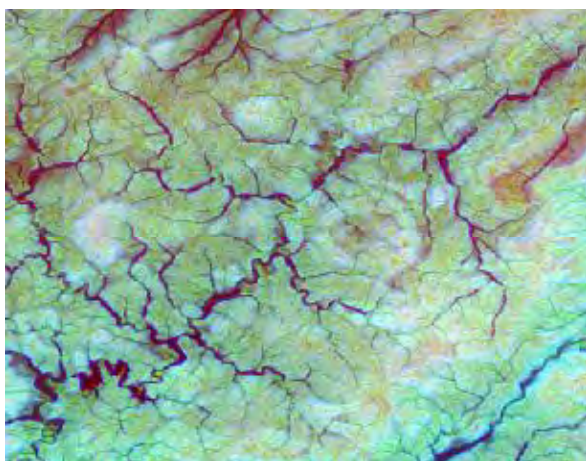
Рис. 3.5. Фрактальная гексагональная структура линейных элементов на северо-западе Корейского полуострова. Синтезированные цвета
