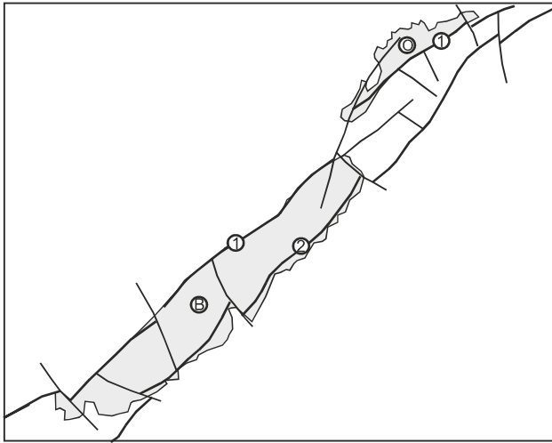
Рис. 3.8.5. Хинганский (1) и Амгуньский (2) разломы, Верхнеамгуньская (В) и Омогуньская (О) впадины
