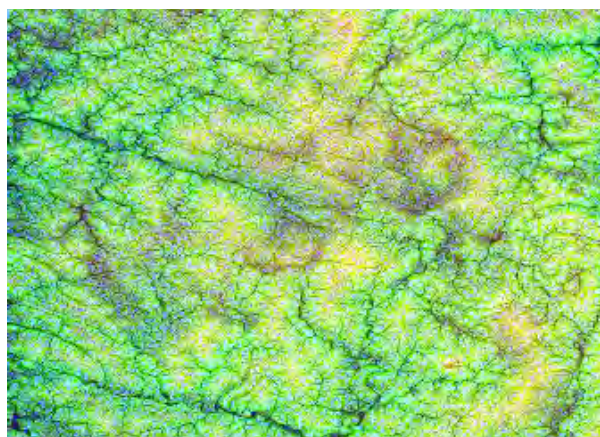
Рис. 3.6. Гексагональная структура, расположенная к югу от показанной на рис. 3.6, в другом сочетании цветов. Рядом просматриваются и другие шестиугольники. Прекрасно выражены линейные элементы северо-западного и северо-восточного простираний, образующие почти правильную квадратную сеть.
