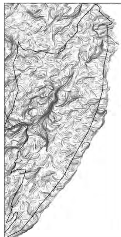
Рис. 3.5.5. Линии вытянутости роз-диаграмм Сихотэ-Алинской складчатой системы
