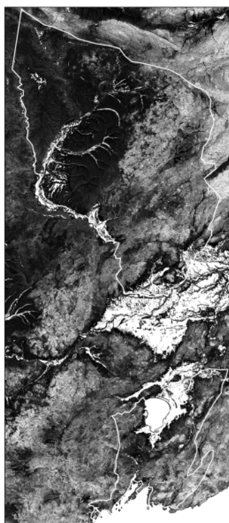
Рис. 3.6.2. ЦМР Буреинского и Ханкайского массивов, обработанная расчетом модуля градиента рельефа
