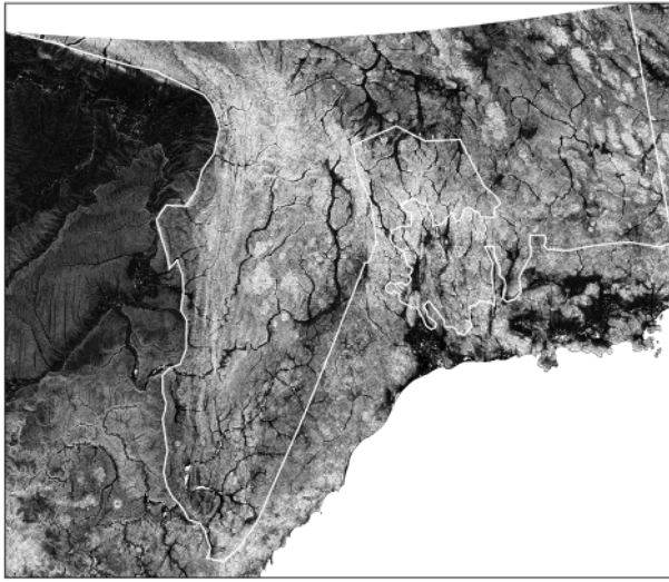
Рис. 3.3.3. Обработанная ЦМР Верхояно-Колымской складчатой системы
