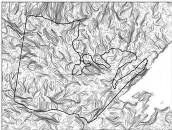
Рис. 3.1.2. Линии вытянутости роздиаграмм линеаментов Алдано-Станового щита
