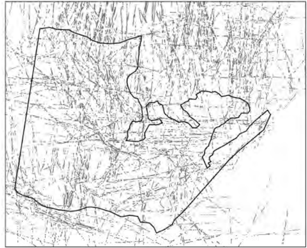
Рис. 3.1.3. Рисунок линеаментов Алдано-Станового щита
