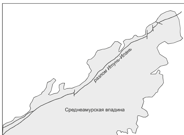
Рис. 3.8.6. Разлом Итунь-Илань и Среднеамурская впадина
