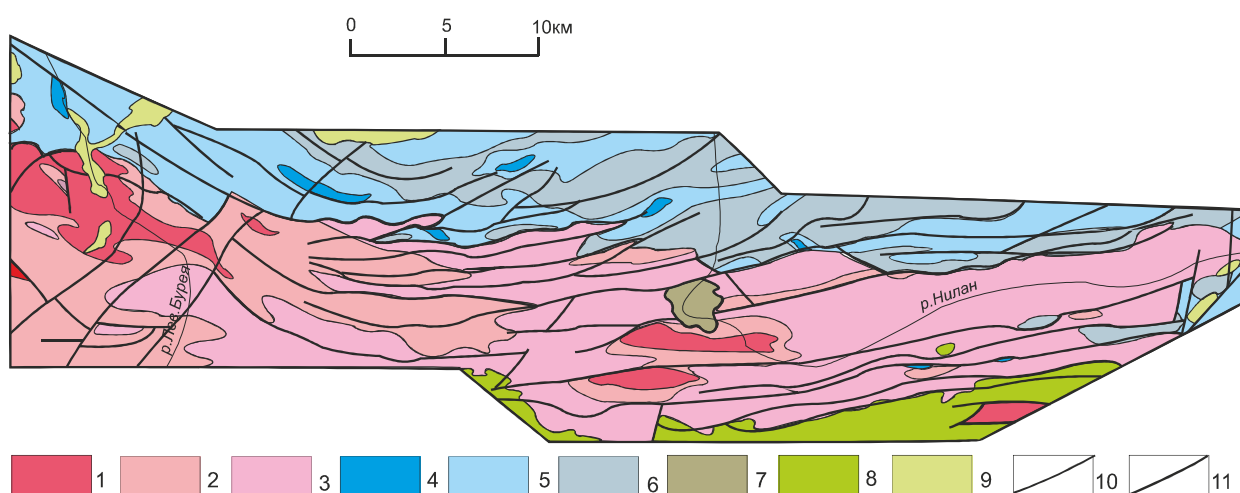
Рис. 4.4. Фрагмент карты тектоноформаций зоны Пауканского глубинного разлома в бассейнах рр. Прав. Бурея и Нилан (по В.Ю. Забродину, 1989 г., с упрощениями).
