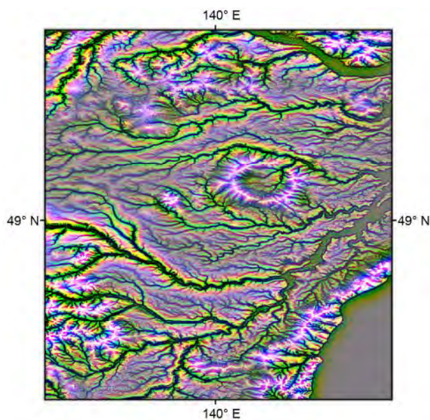
Рис. 2.6.3. Пример выделения кольцевой структуры в Восточно-Сихоте-Алинском вулcano-плутоническом поясе.
