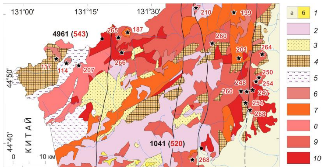
Рис. 3. Схема геологического строения северо-западной части Ханкайского массива
