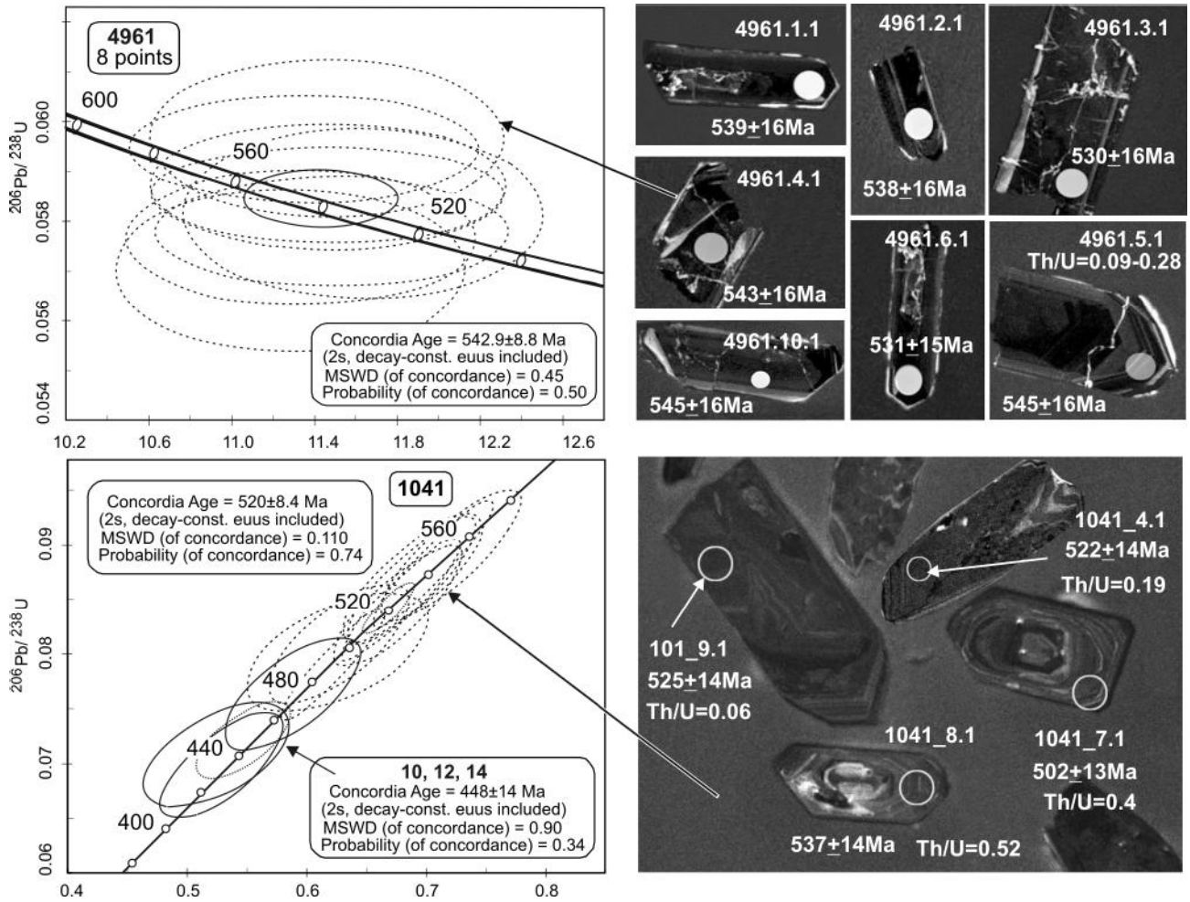
Рис. 6. Катодолуминисцентные изображения цирконов и U-Pb диаграммы с конкордией.
