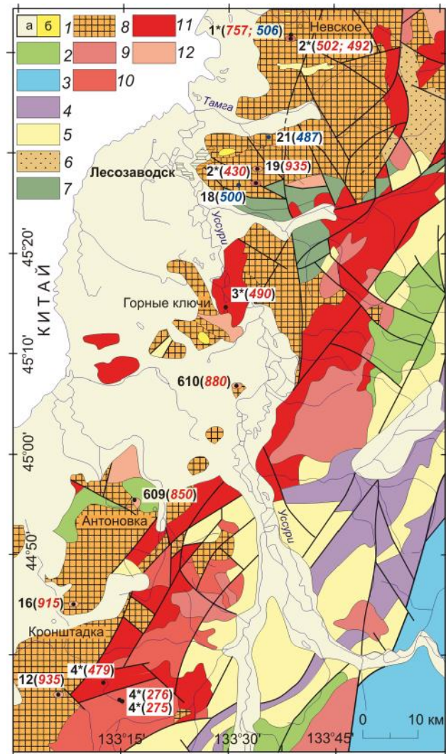
Рис. 2. Схема геологического строения северной части Ханкайского массива (по [3], с изменениями).
