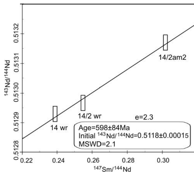
Рис. 7. Sm-Nd изохрона по амфиболу и валовым пробам из габбро и перидотитов дмитриевского комплекса.
