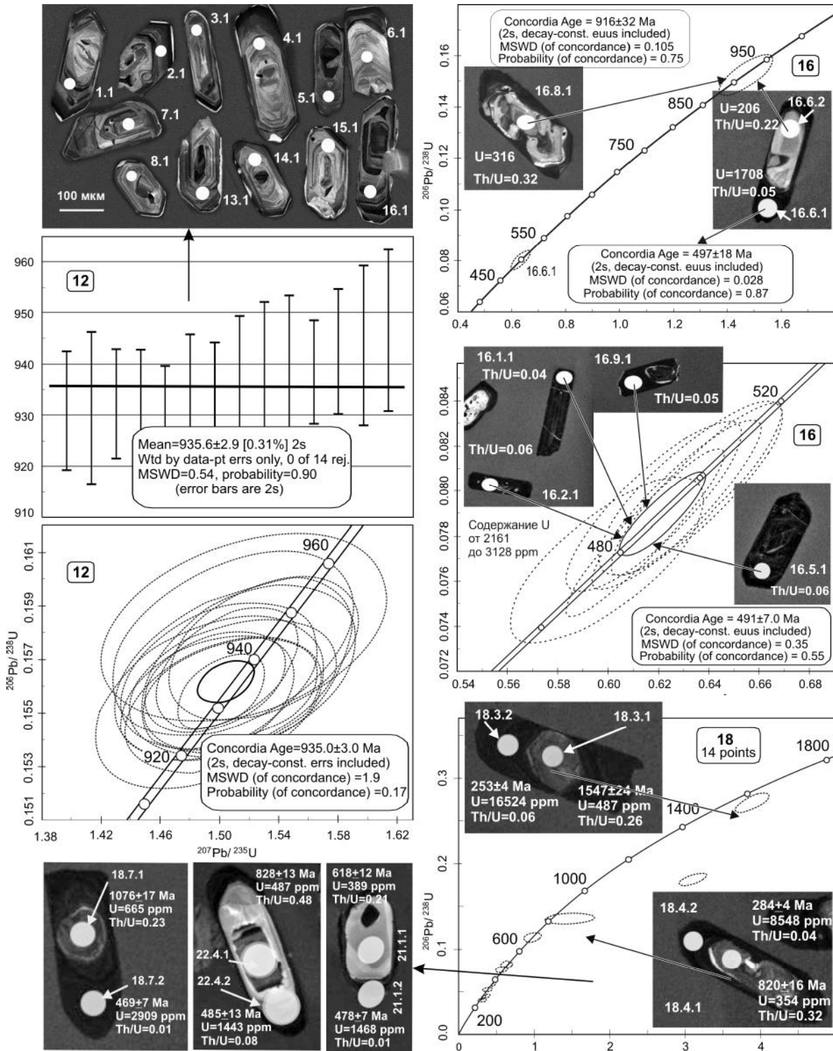
Рис. 4. Микрофотографии типичных кристаллов циркона в режиме КЛ, гистограмма возрастов и U-Pb диаграмма с конкордией по цирконам (обр. 12), КЛ изображения цирконов и диаграммы с конкордией для цирконов из двупироксенового гранулита (обр. 16), гнейса (обр. 18), метамонцитита (обр. 21)).
