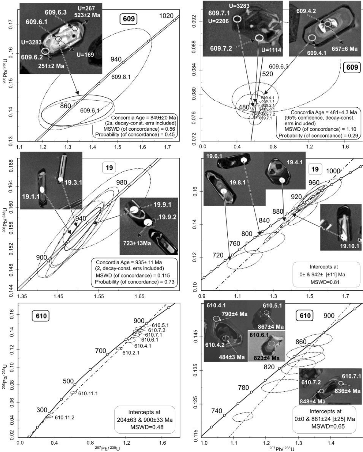
Рис. 5. КЛ изображения цирконов с местами анализов в ядрах и оболочках и диаграммы с конкордией для цирконов из гнейсогранитов (обр. 19, 609, 610).
