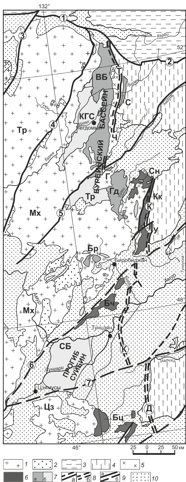
Рис. 1. Структурная схема зоны сочленения Буреинско-Цзяму-сы-Ханкайского массива и Сихотэ-Алинской складчатой системы (по [5] с дополнениями и изменениями).
