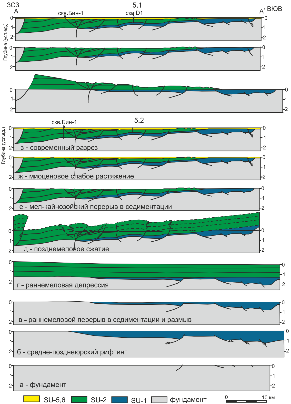
Рис. 5. История эволюции прогиба Суйбин на примере разреза сейсмического профиля А-А' [21]: 1 – сбалансированный разрез по поверхности тектоно-стратиграфического комплекса SU-1; 2 – реконструкция осадконакопления и деформаций.
