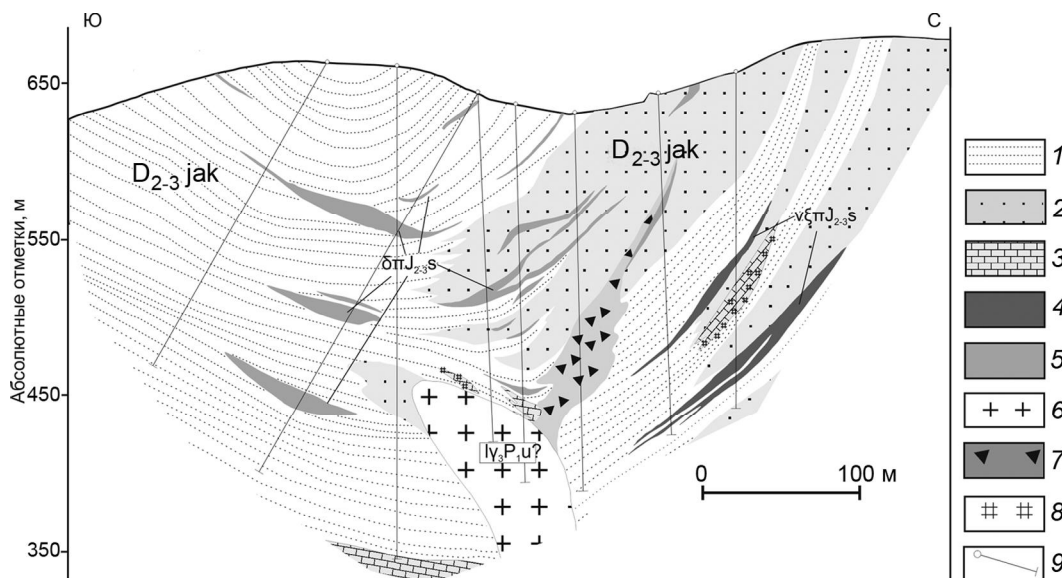
Рис. 3. Схематический геологический разрез месторождения Серебряное (составлен на основе данных ООО «Востокгеология»).
