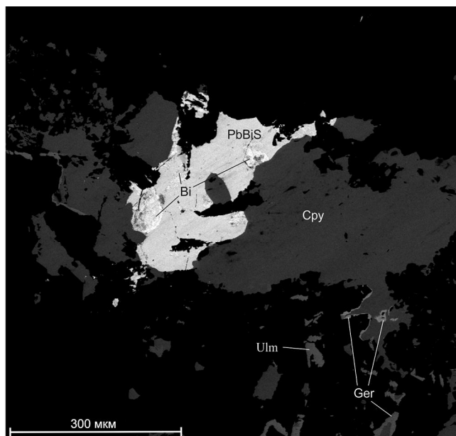
Рис. 5. Характерное взаимоотношение висмутовых минералов с халькопиритом (снято в отраженных электронах).
