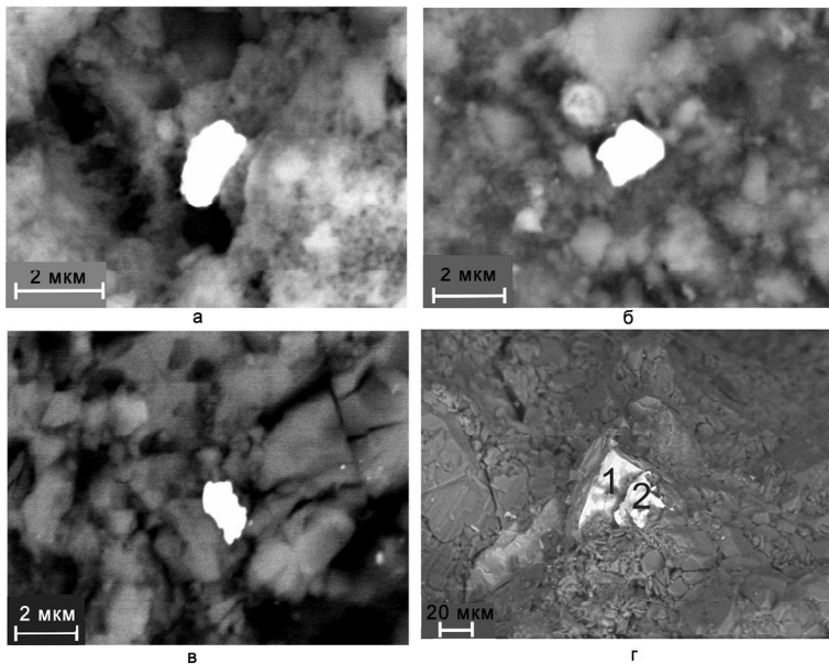
Рис. 5. Рудные минералы в продуктивных тонкозернистых и микрозернистых кварцах Покровского месторождения.
