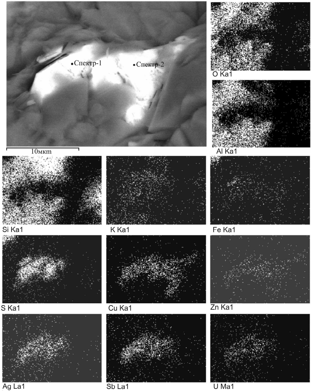
Рис. 6. Рентгеновская картограмма срастания фрейбергита с интерметаллидом Cu и Zn (правая часть сrostка) в алюмо-кремниво-калиевом метасоматите на границе с кварцем.
