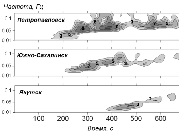
Рис. 5. СВАН-диаграммы вертикальной компоненты сейсмического сигнала при землетрясении 13.01.2007 на станциях “Петропавловск”, “Южно-Сахалинск” и “Якутск”. Спектры нормированы на значение скорости 4 мм/с (“Петропавловск” – 6 мм/с), отвечающее уровню 10, изолинии проведены через 2 дБ.
