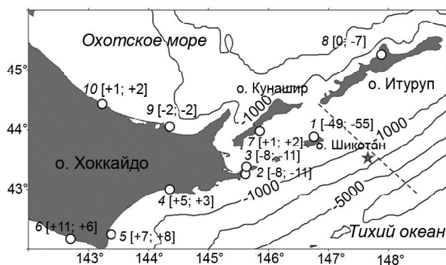
Рис. 1. Положение мареографных станций на Южных Курильских островах (1 – Малокурильское, 7 – Южно-Курильск, 8 – Курильск) и северо-восточной части о. Хоккайдо (2 – Ханасаки, 3 – Немуроко, 4 – Кусиро, 5 – Токачиико, 6 – Уракава, 9 – Абасири, 10 – Момбецу).
