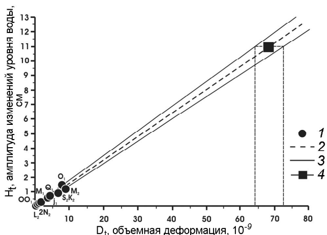
Рис. 2. Зависимость выделенных амплитуд приливных волн суточной и полусуточной групп в изменениях уровня воды в скважине ЮЗ-5 ( H_t ) от теоретических величин приливной объемной деформации D_t .
