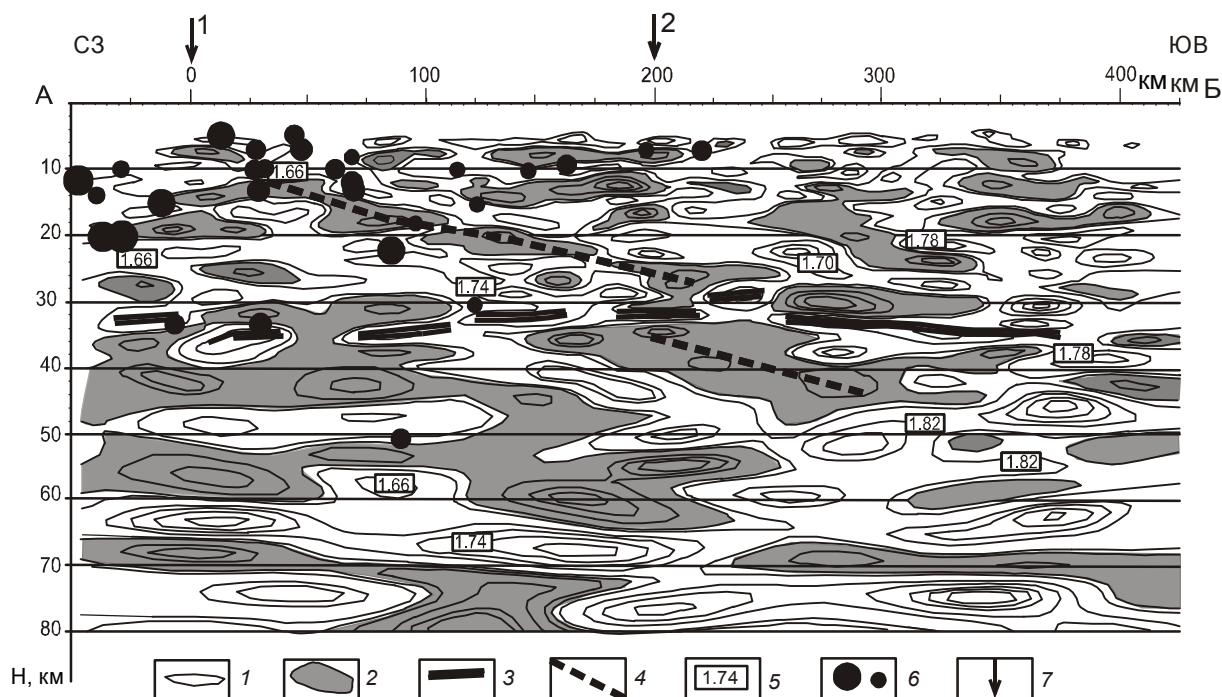
Рис. 5. Сейсмический разрез (МОВЗ) через Среднеамурский бассейн.
