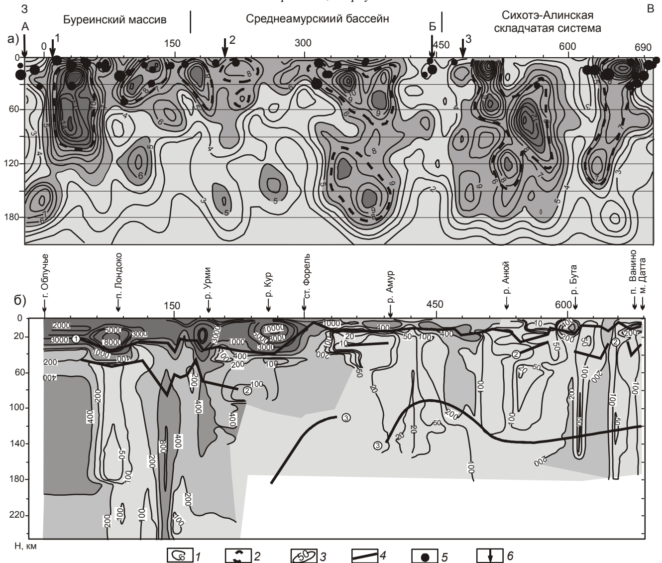
Рис. 6. Результаты глубинных геофизических исследований по профилю Облучье – мыс Датта: а – сейсмический (МОВЗ) разрез, б – геоэлектрический (МТЗ) разрез, по [8].
