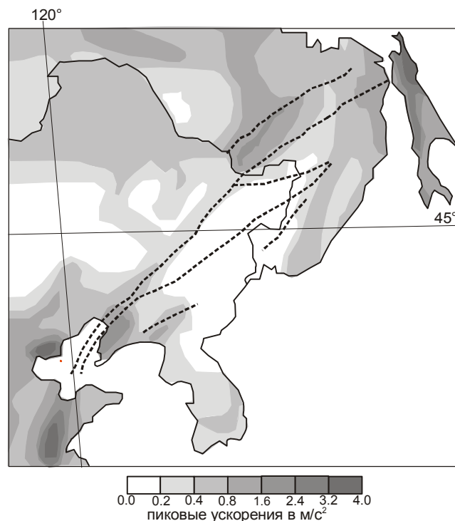
Рис. 8. Сейсмоопасные зоны Тан-Лу-Охотской рифтовой системы, по [44].
